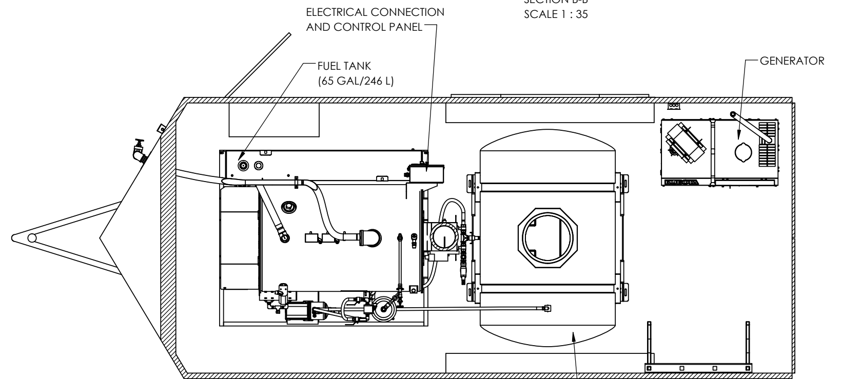
SECTION A-A SCALE 1 : 35
