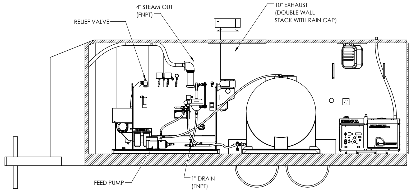
SECTION B-B SCALE 1 : 35
